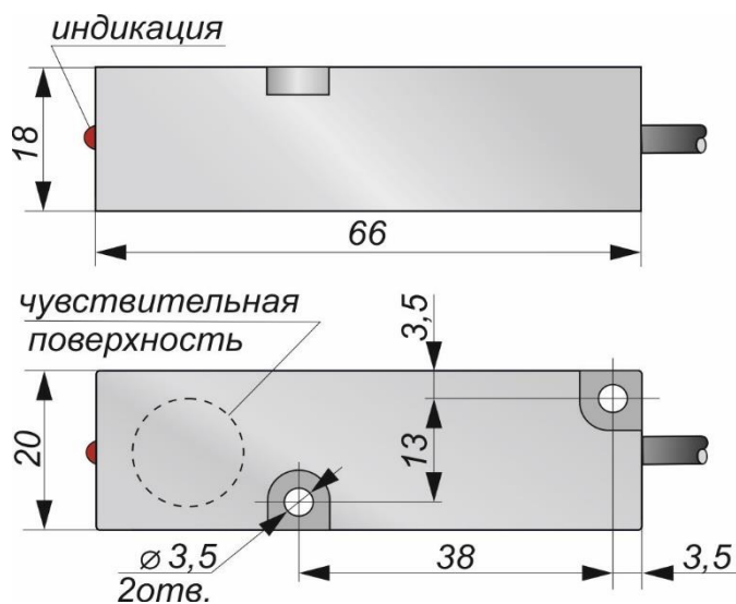
Габаритный чертеж
